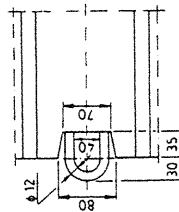
SZCZEGÓL "A"
